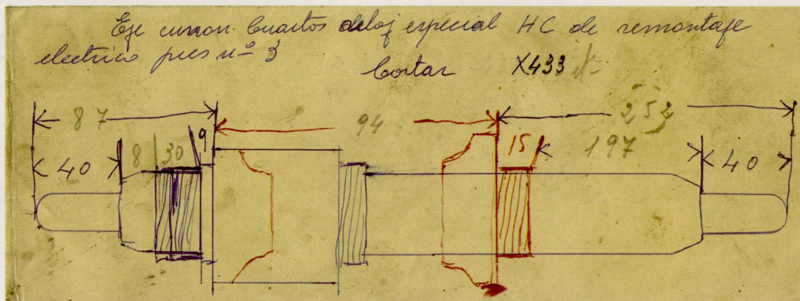
Fitxes de croquis de peces (pàg. anterior i actual)
