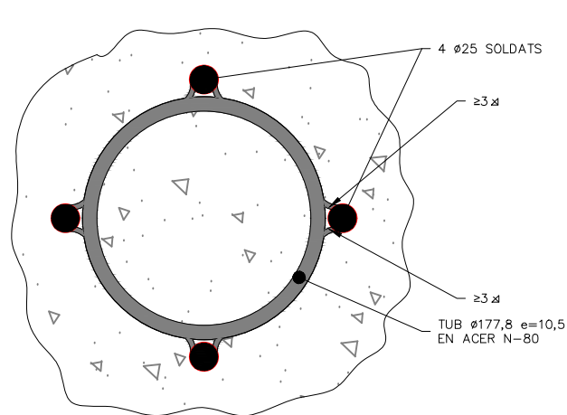
SECCIÓ II
