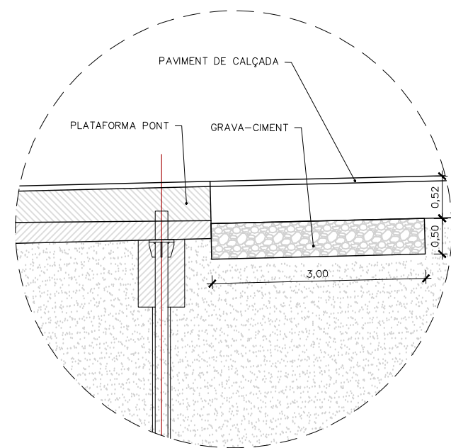
DETALL 1 ESCALA 1/75 DIMENSIONS EN M
