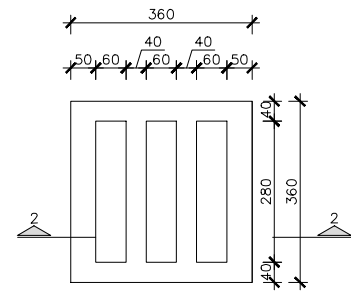
PLANTA REIXETA
