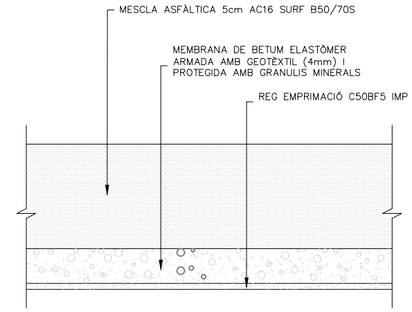
IMPERMEABILITZACIÓ
