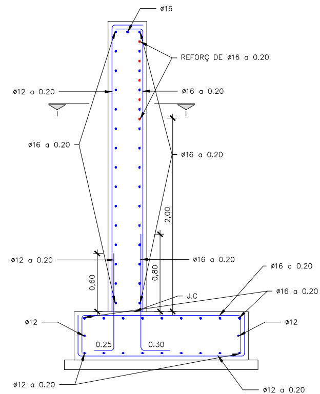
MUR TIPUS A H \leq 3m
