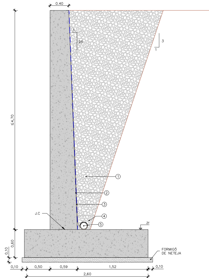
MUR TIPUS C H≤4.70m
