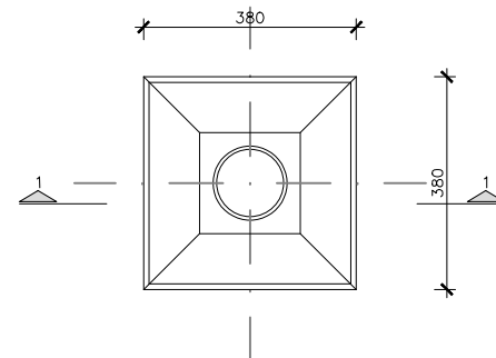
PLANTA EMBORNAL
