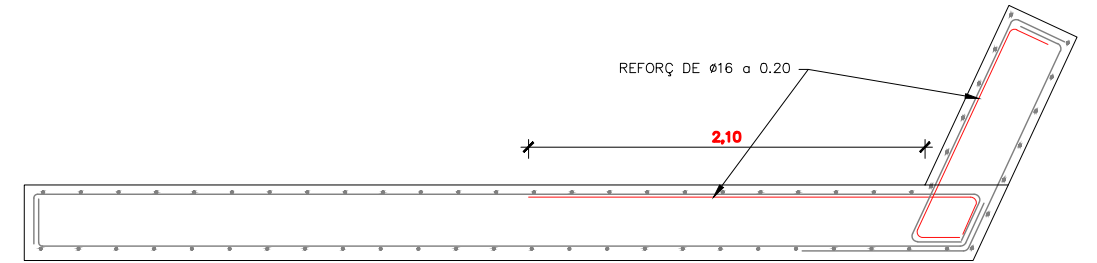
SECCIÓ I ARMAT DE REFORÇ ESCALA 1/40 DIMENSIONS EN M
