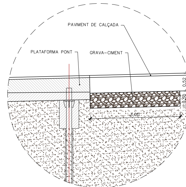
DETALL 1 ESCALA 1/75 DIMENSIONS EN M
