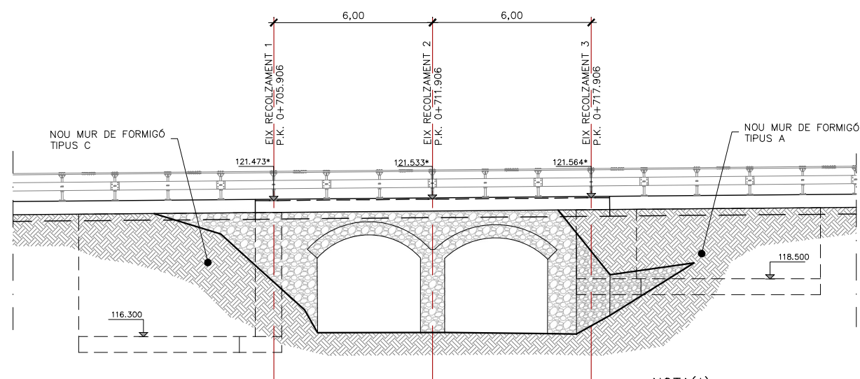
ALÇAT
