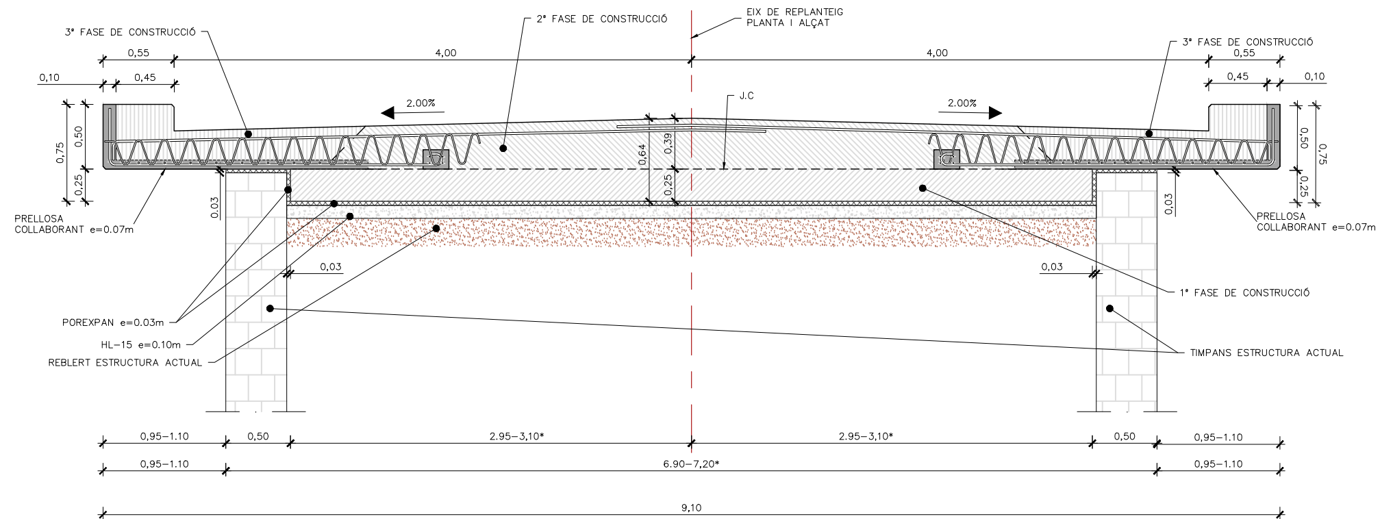
SECCIÓ TRAM CENTRAL
