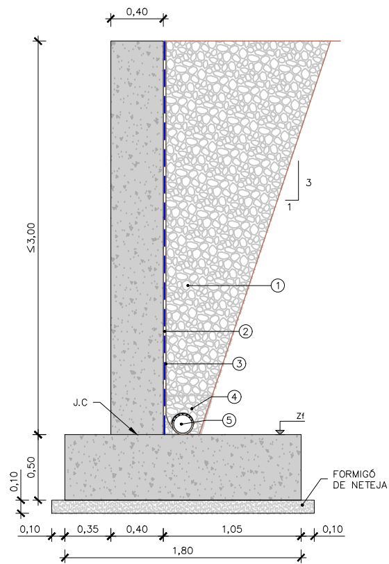
MUR TIPUS A H≤3m
