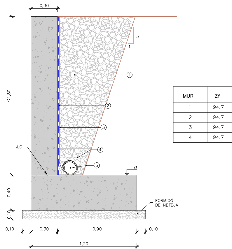
MUR TIPUS D H≤1.80m
