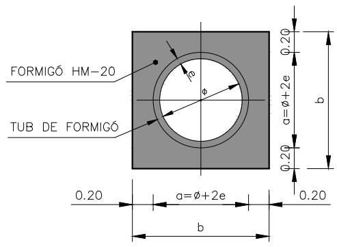
SECCIÓ B-B ESCALA = 1/50
