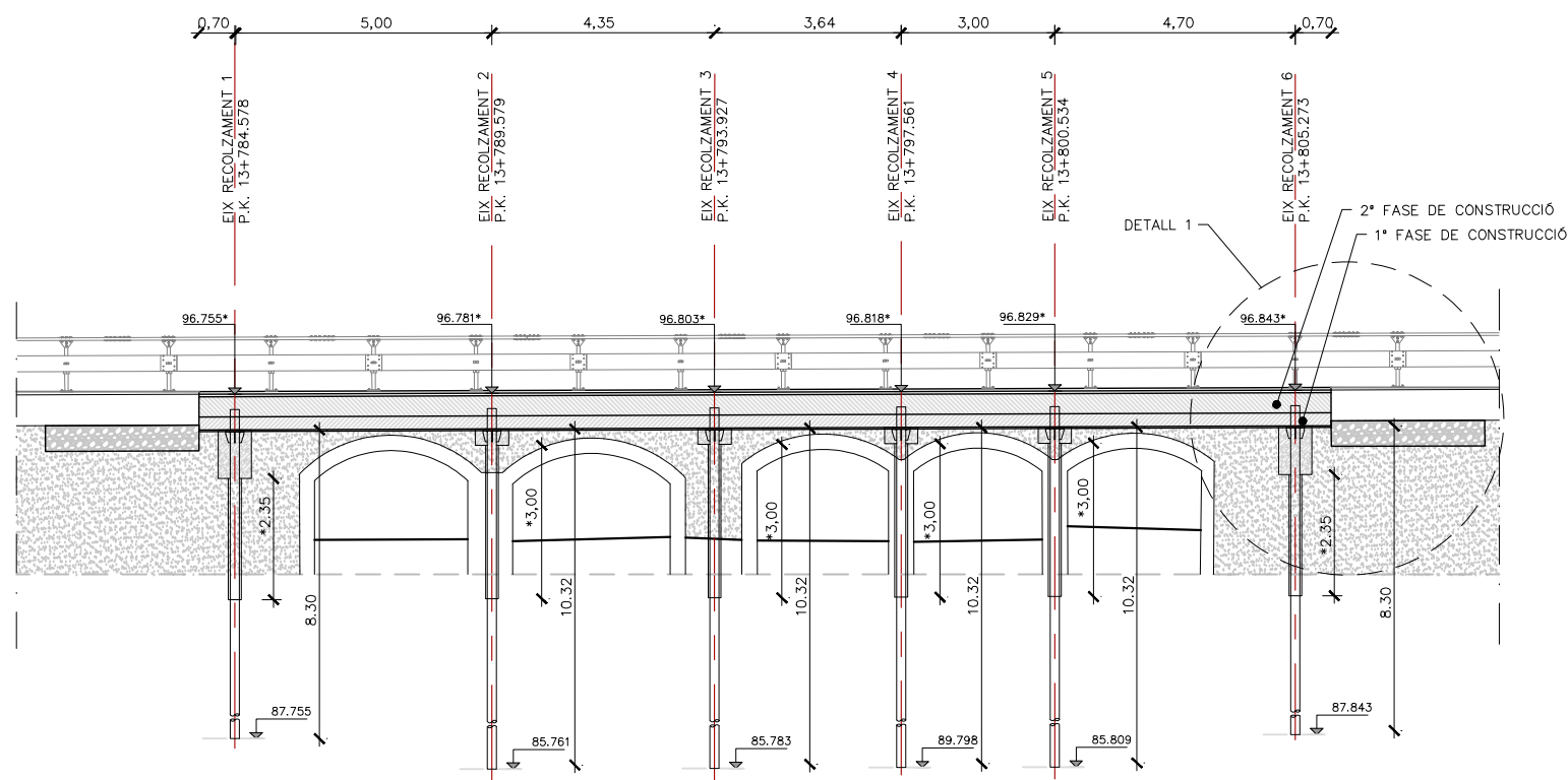
SECCIÓ LONGITUDINAL ESCALA 1/150 DIMENSIONS EN M
