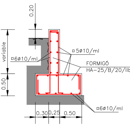
ALETES SECCIÓ C-C
