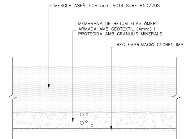
IMPERMEABILITZACIÓ
