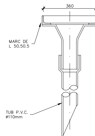
SECCIÓ 1
