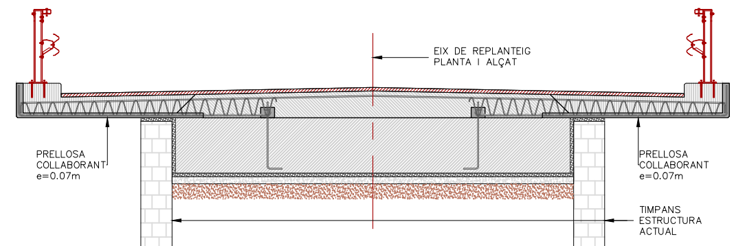
SECCIÓ TIPUS I 4ª FASE ESCALA 1/75 DIMENSIONS EN M
