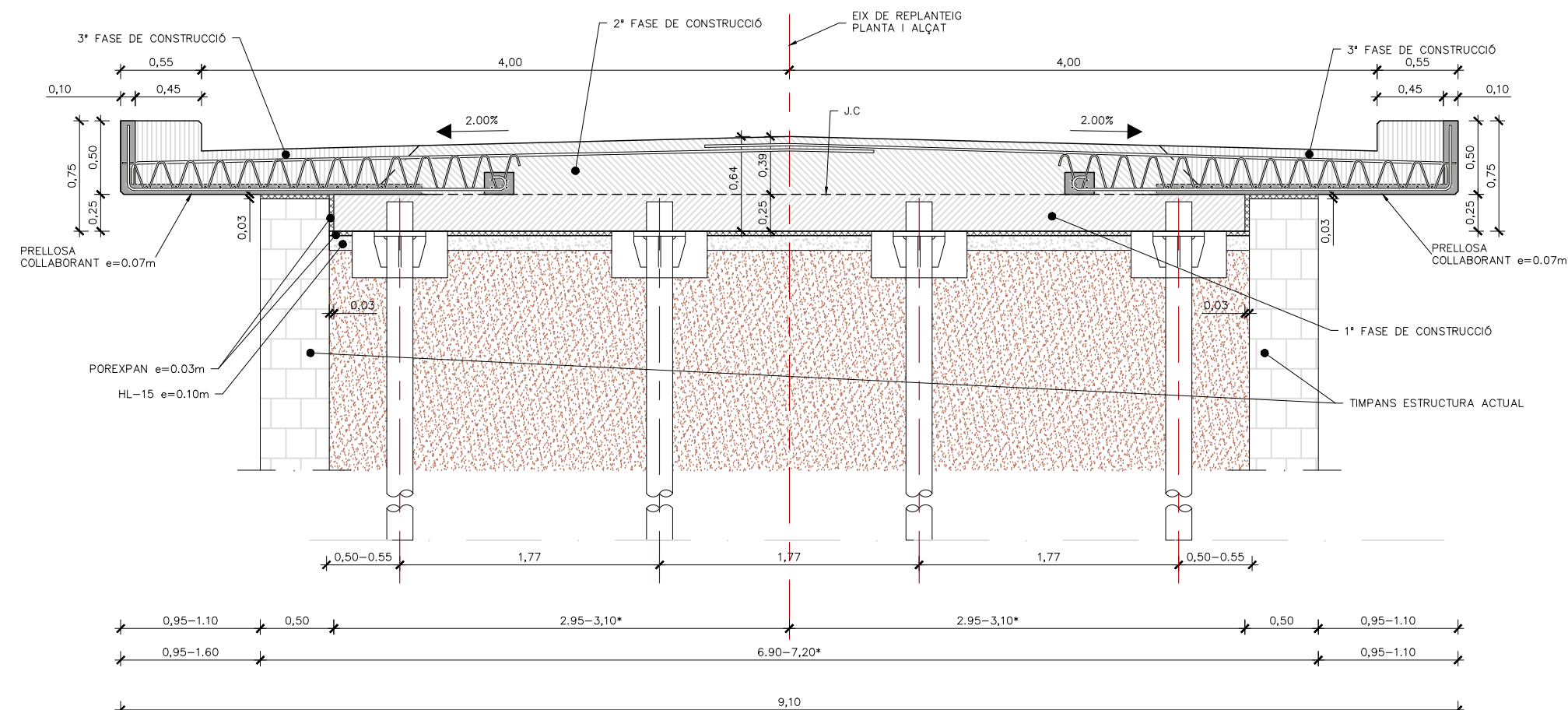
SECCIÓ TRAM RECOLZAMENT
