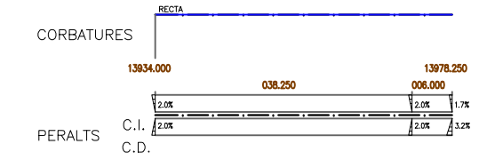
EIX 3
