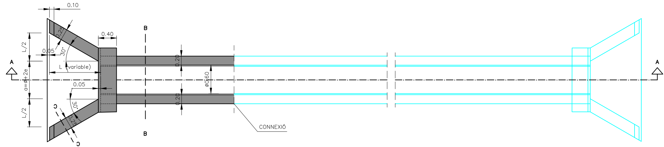
PLANTA ESCALA = 1/50
