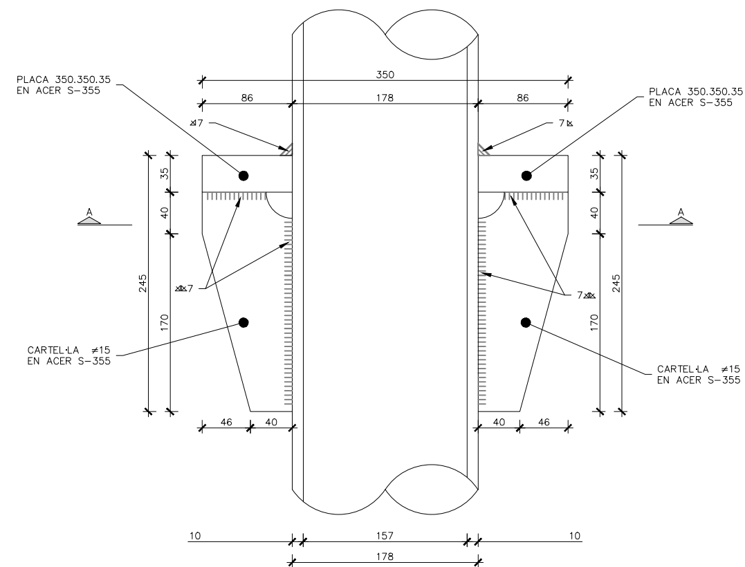
SECCIÓ B
