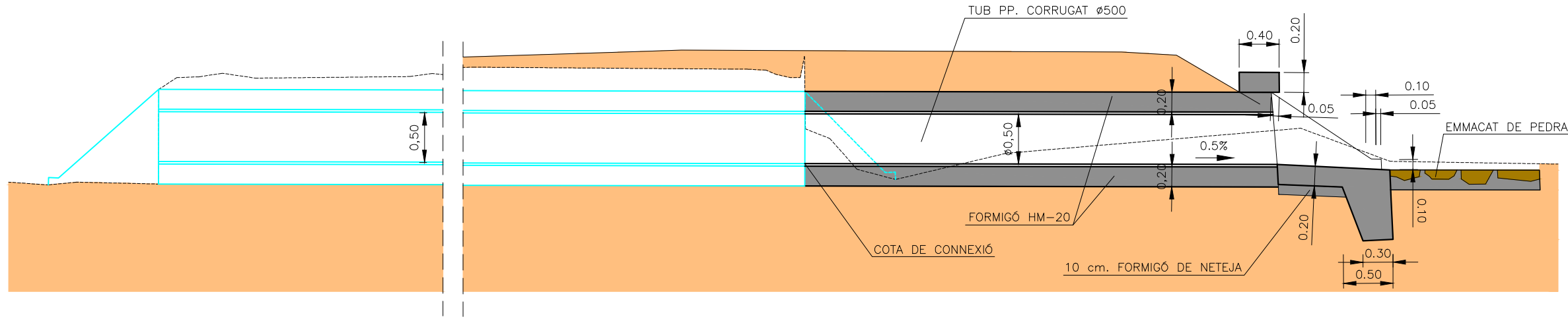
SECCIÓ A-A ESCALA = 1/50
