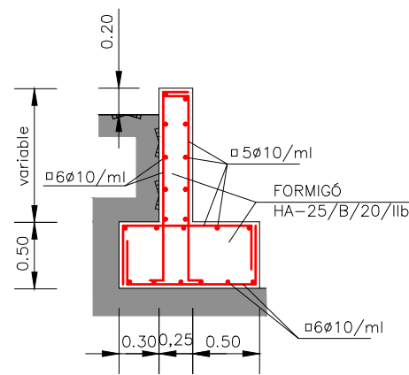
ALETES SECCIÓ C-C
