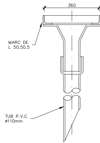
SECCIÓ 1
