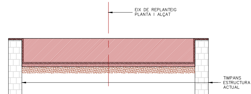
SECCIÓ TIPUS I 1ª FASE ESCALA 1/75 DIMENSIONS EN M
