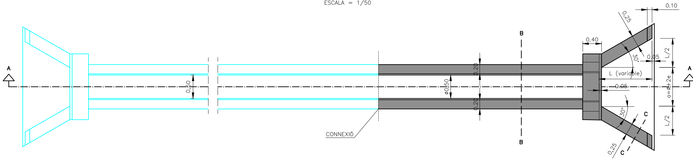
PLANTA ESCALA = 1/50
