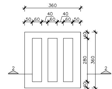
PLANTA REIXETA
