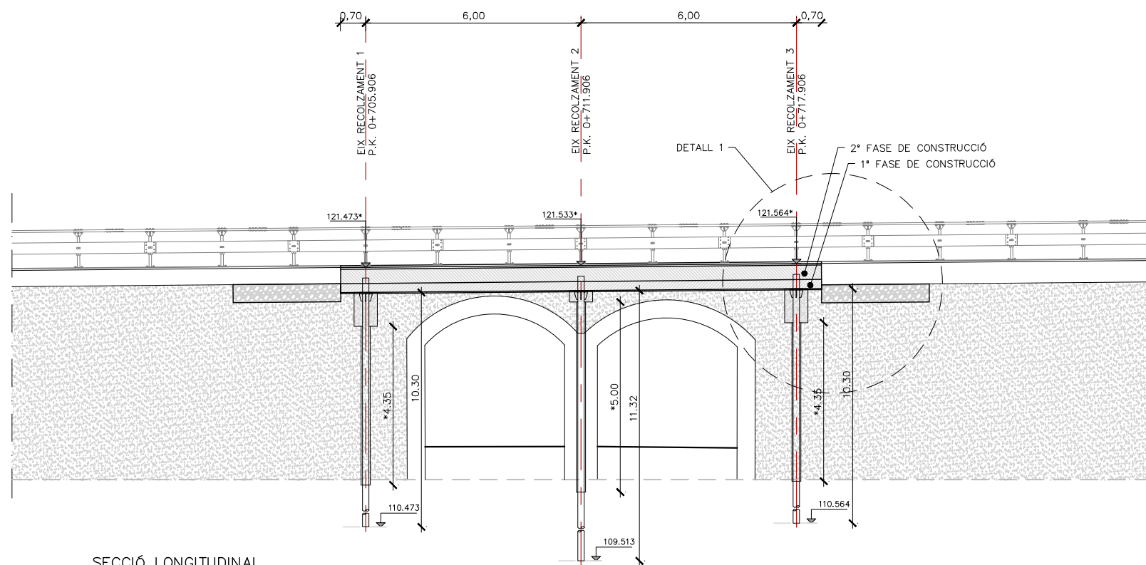
SECCIÓ LONGITUDINAL ESCALA 1/150 DIMENSIONS EN M
