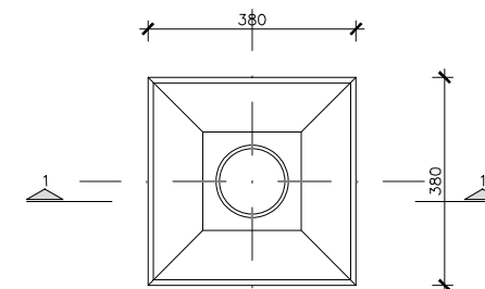
PLANTA EMBORNAL
