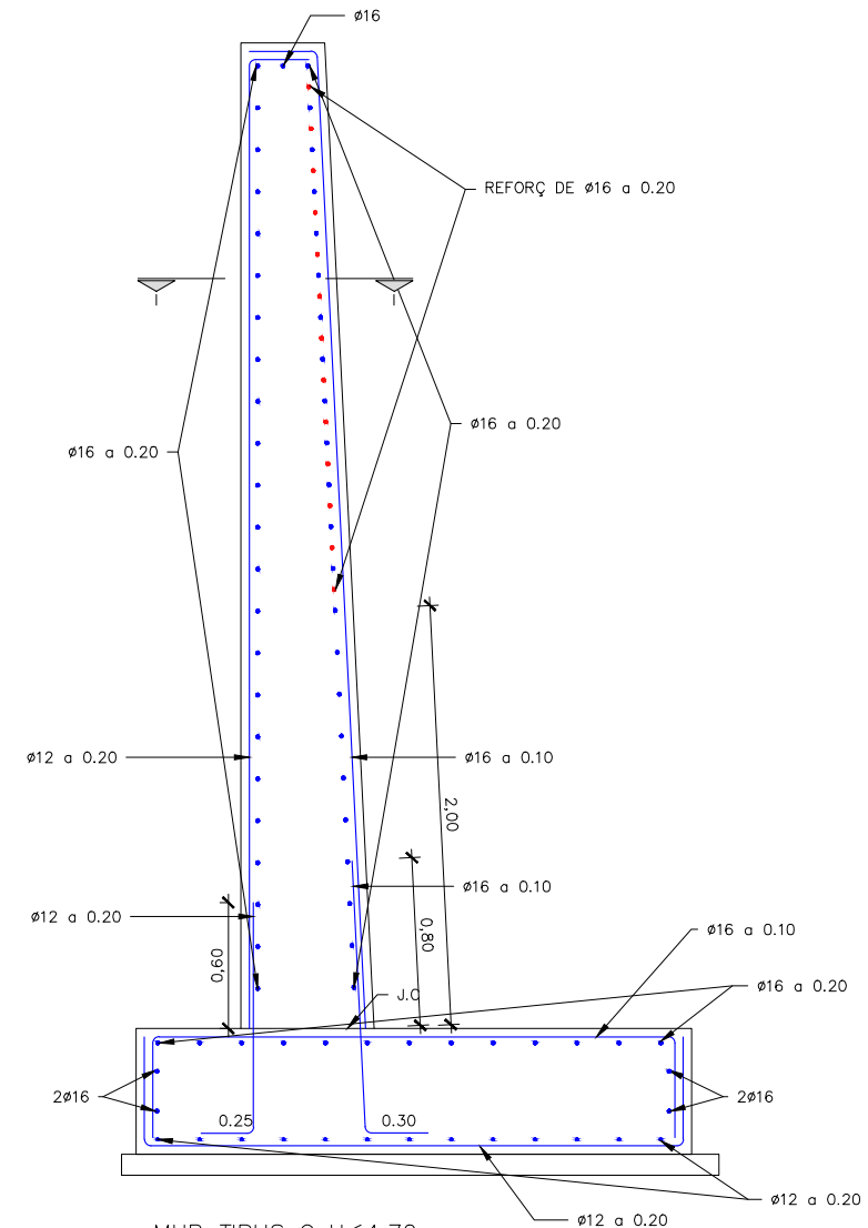
MUR TIPUS C H \leq 4.70m
