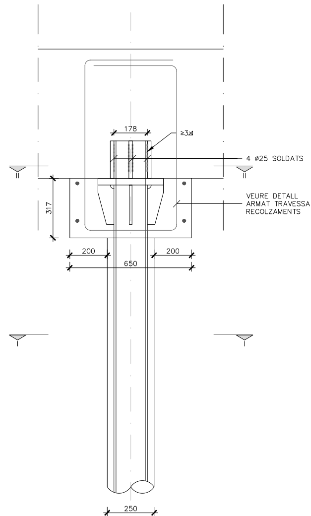
DETALL MICROPILONS
