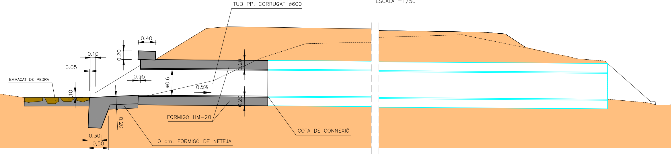
SECCIÓ A-A ESCALA = 1/50
