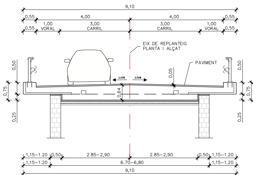
SECCIÓ TRANSVERSAL
