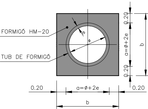
SECCIÓ B-B ESCALA = 1/50
