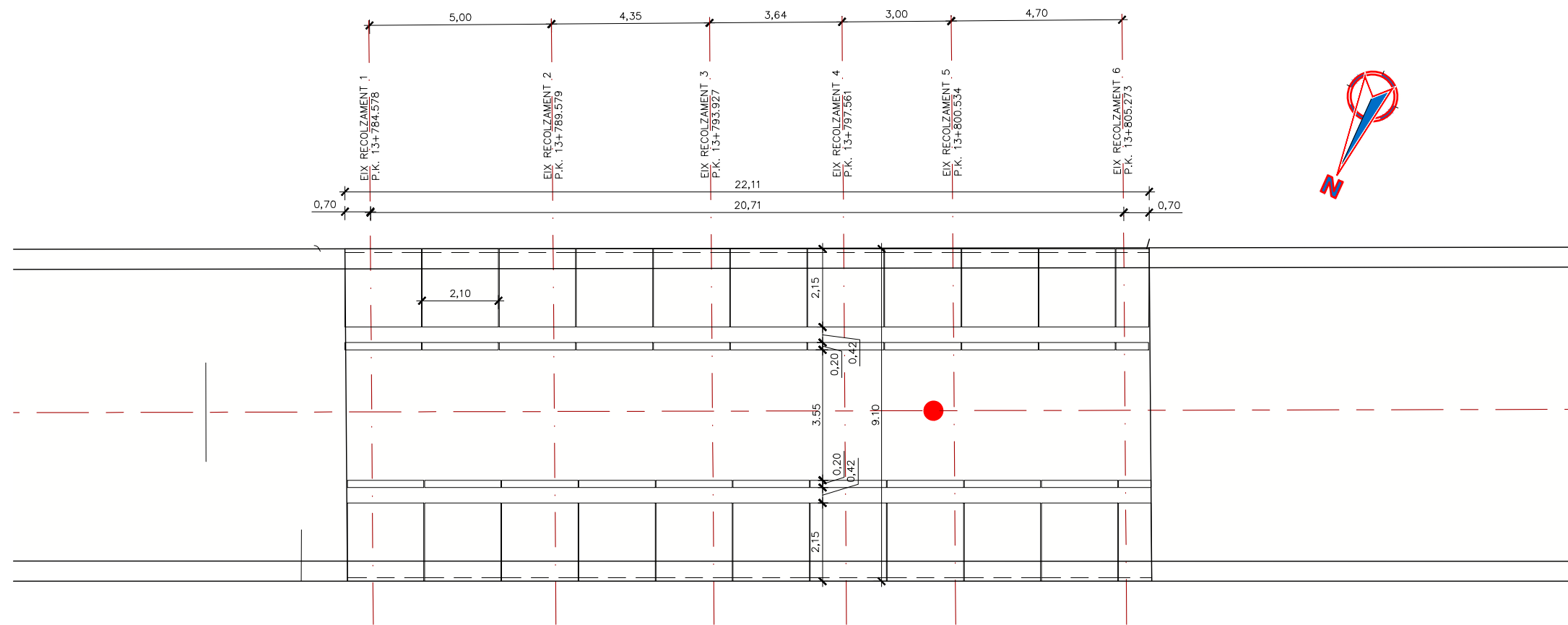
PLANTA GENERAL. PRELLOSES ESCALA 1/150 DIMENSIONS EN M
