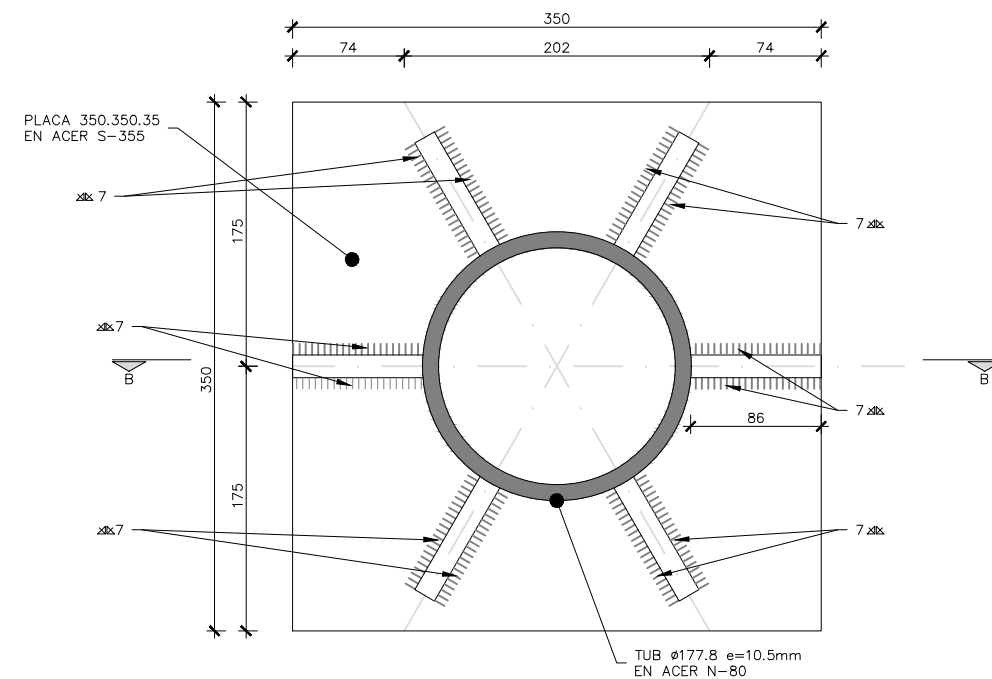
SECCIÓ A
