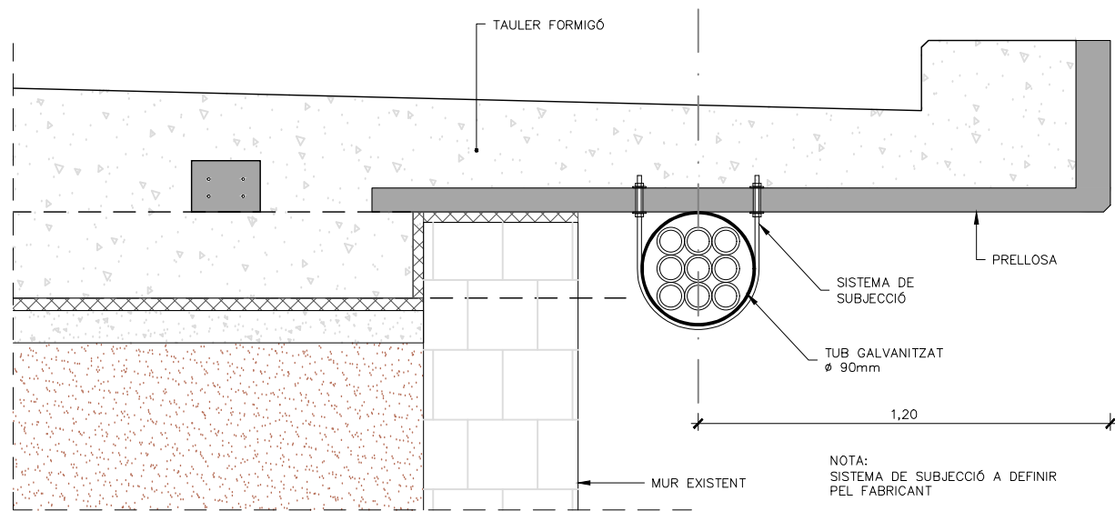
DETALL SUBJECCIÓ FIBRA
